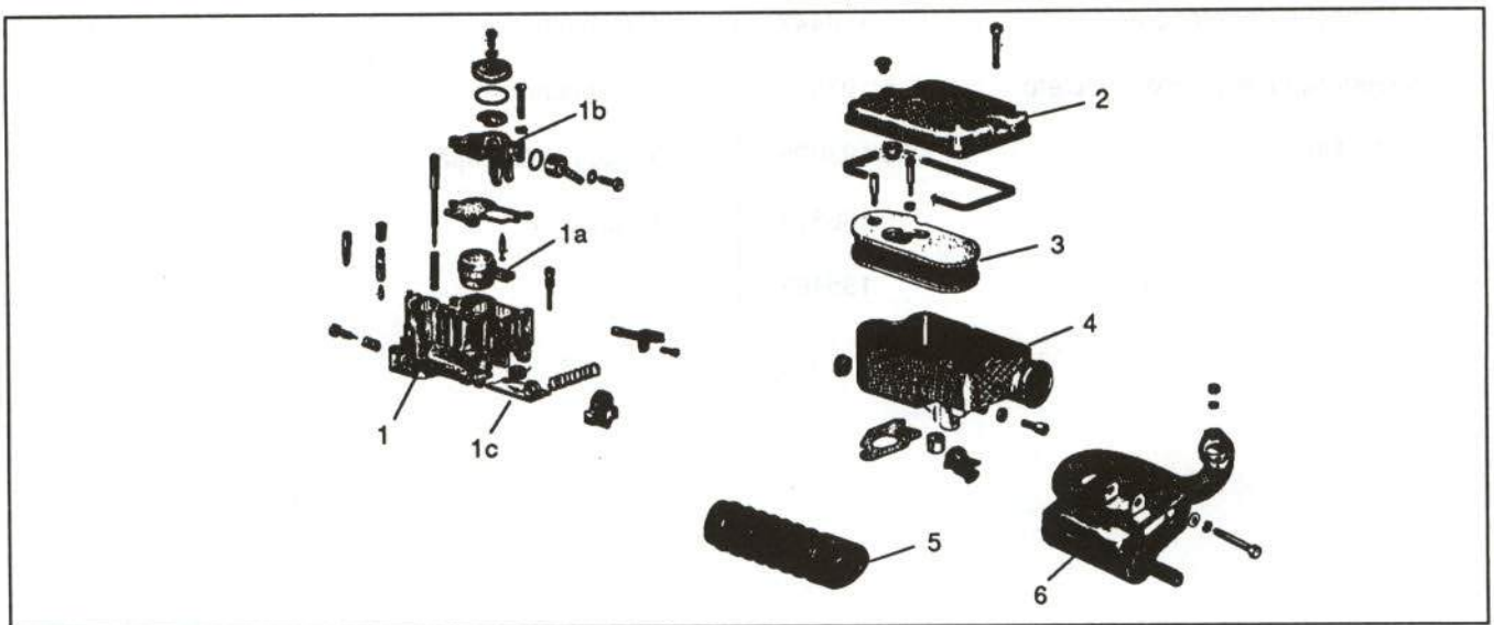
Figura 11. Despiece de admisión y escape
