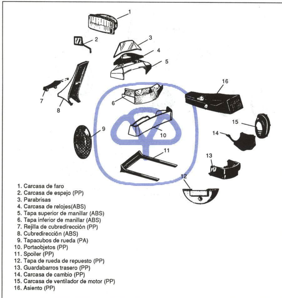
Figura 3.- Piezas de material plástico
