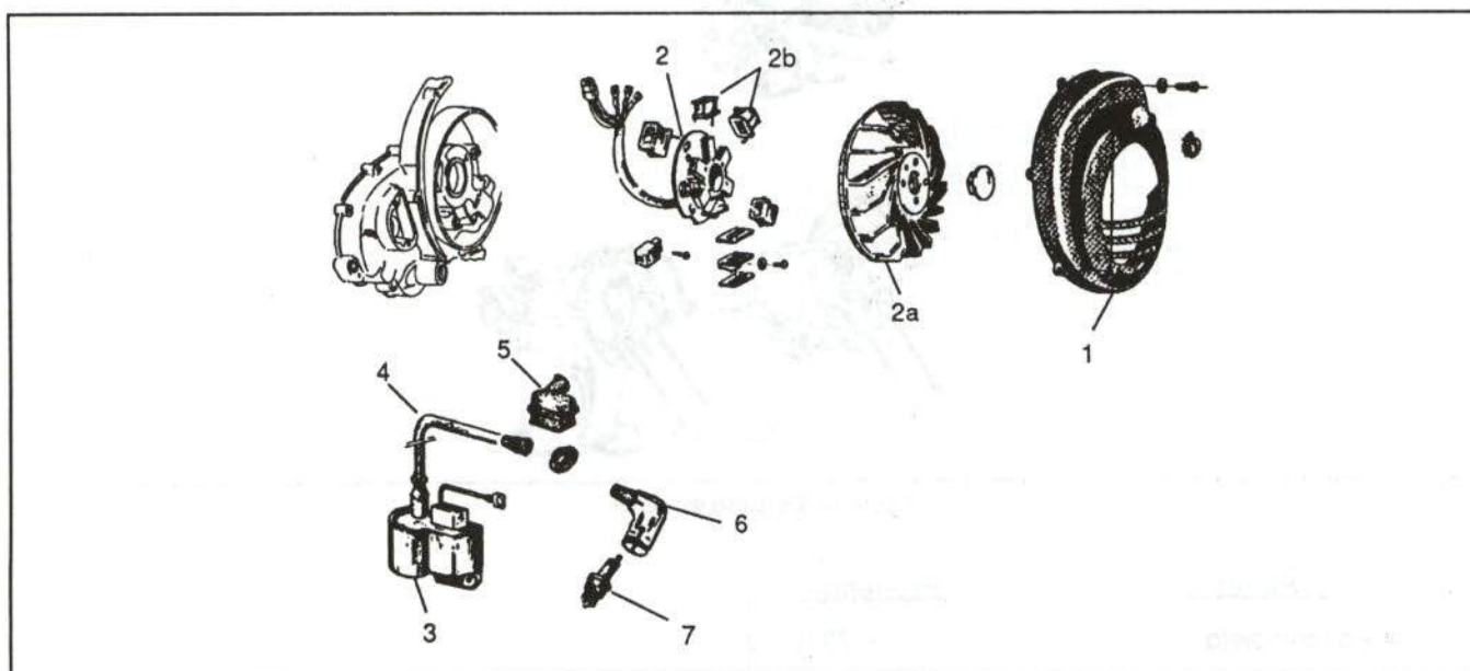
Figura 9c. Despiece del generador
