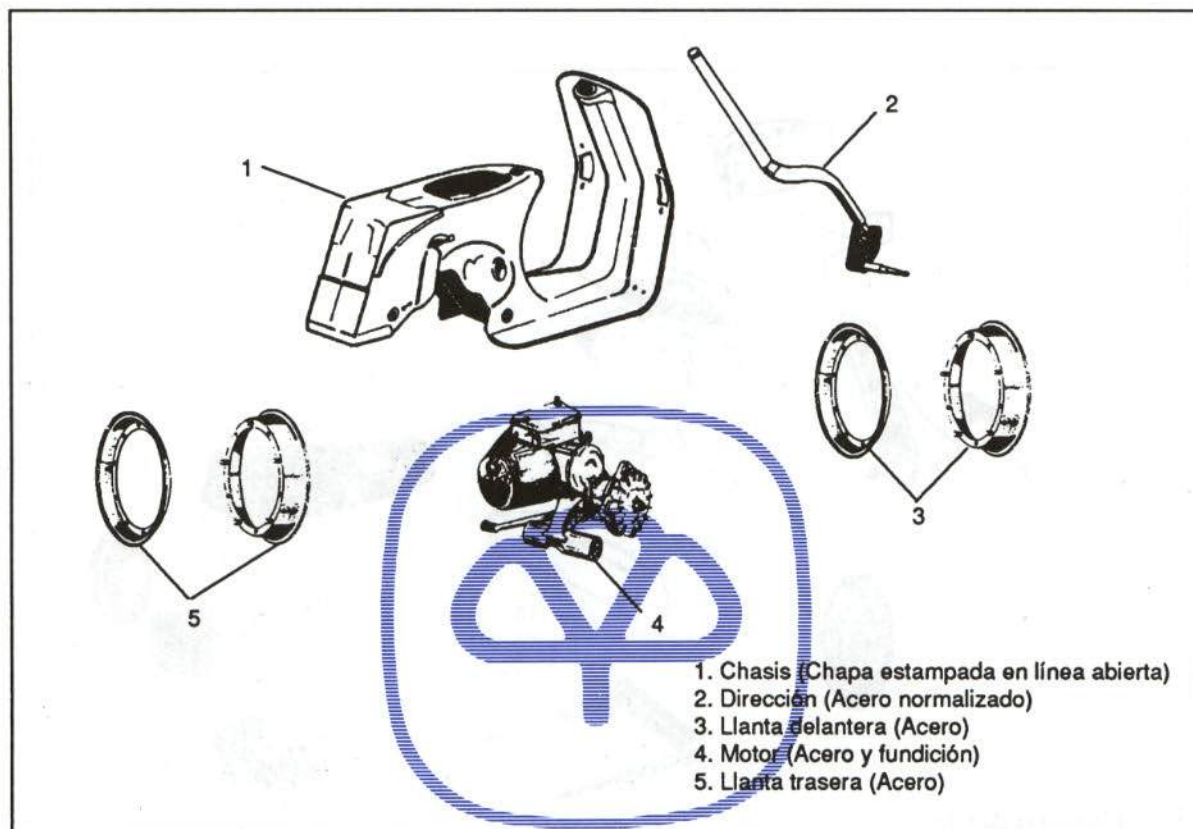
Figura 4.- Piezas de material metálico
