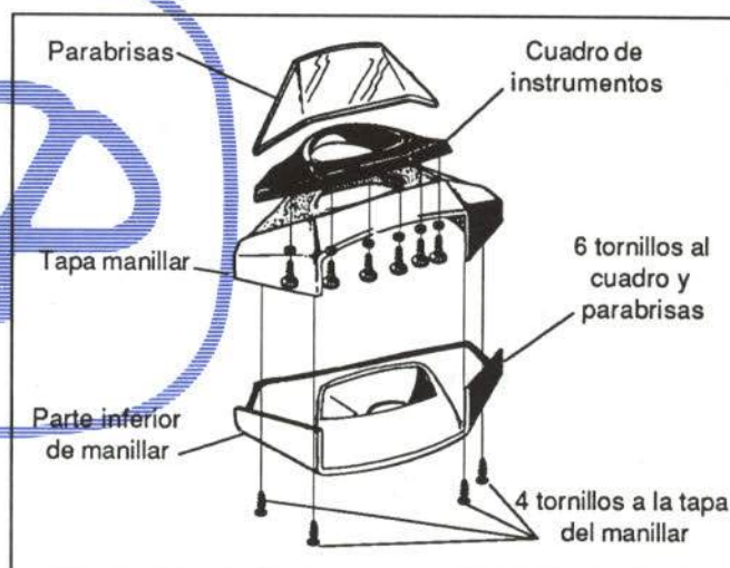
Figura 15.- Unión de la carcasa de cuadro
