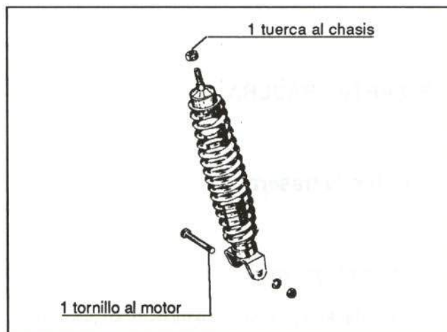
Figura 29.- Fijación del amortiguador trasero
