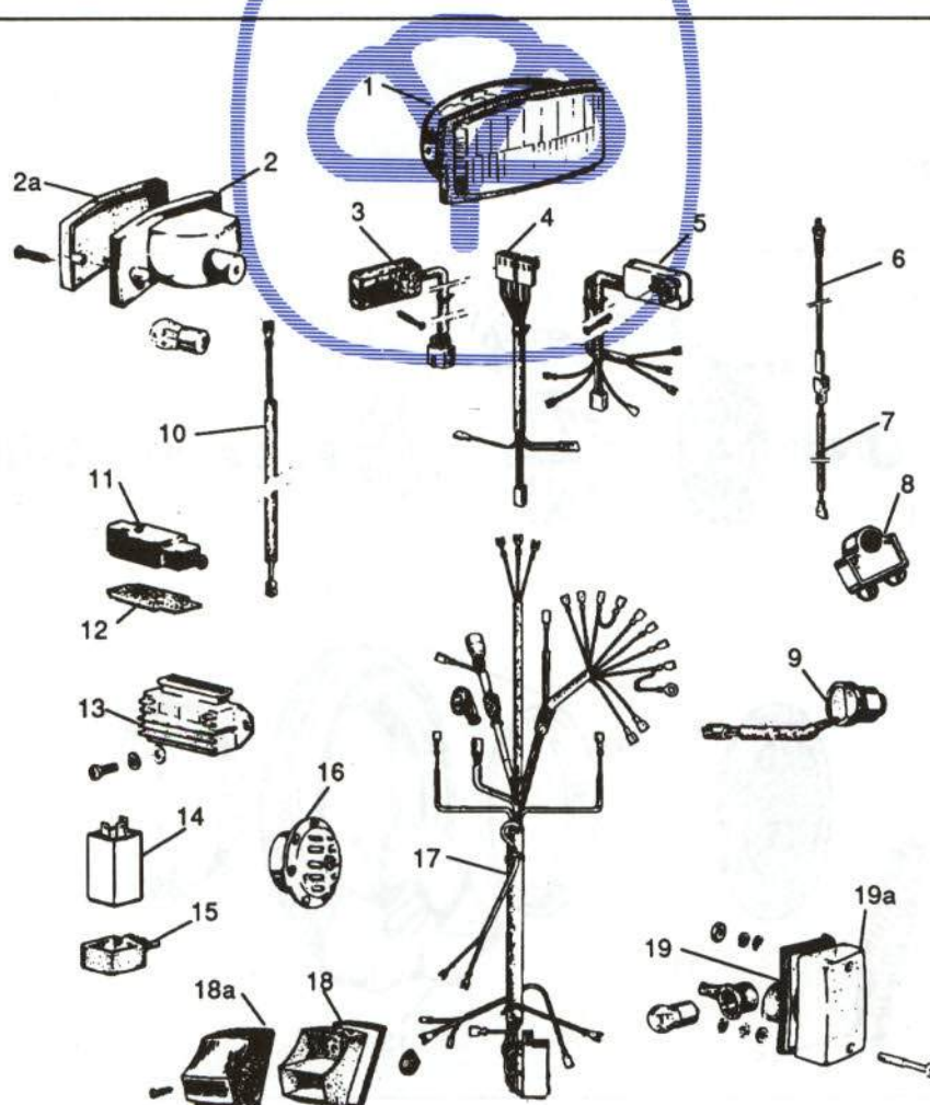
Figura 8.- Despiece de instalación eléctrica
