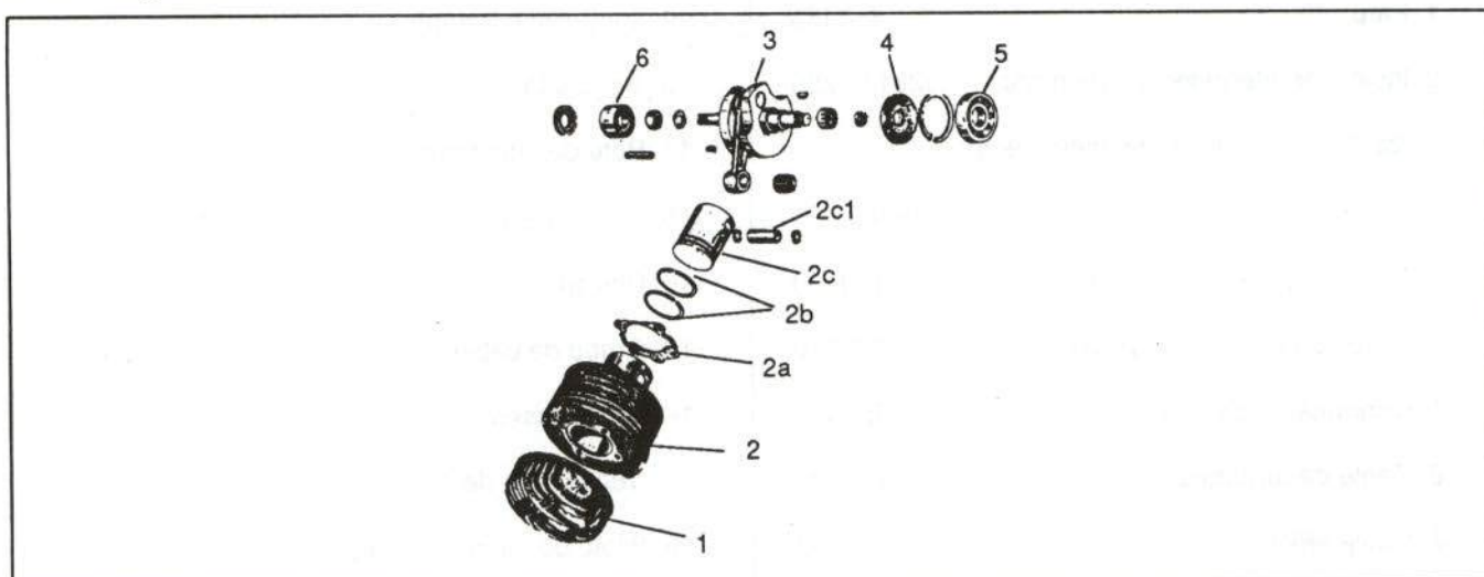
Figura 9b. Despiece del cigüeñal
