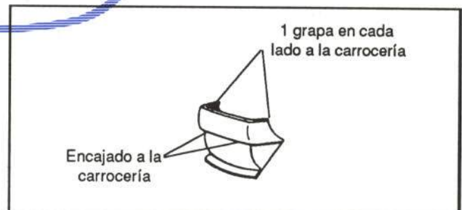
Figura 22.- Fijación del guardabarros trasero
